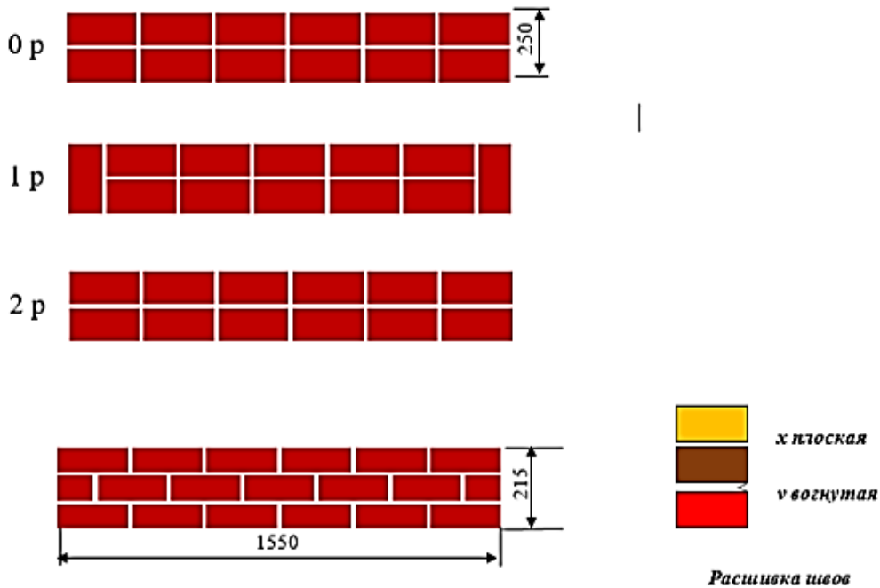
Раскладка кирпича
